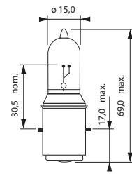
M5 (BA20d)
