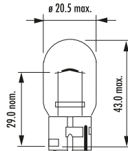
W(Y)21W
