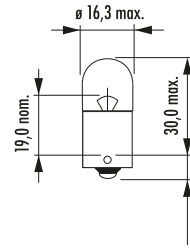
R5W, R(Y)10W, (BA15s)
