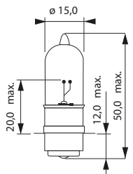
M5 (P15d-25-1)
