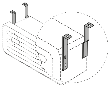
Fixation pour coffre à outils fixation verticale, kit 4 pattes avec vis Ref. 3350102
