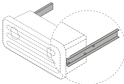
Fixation pour coffre à outils fixation horizontale, kit 2 pattes avec vis Ref. 3350101
