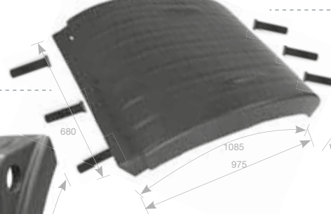
Calotte gauche/droite Ref. 3320037 Ref OE 81664106086
