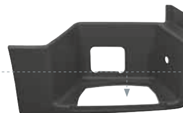
Marche-pied inférieur droit avec trappe Ref. 318560004 Ref OE 81615100798
